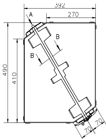
Деталь: уголки для штабелирования
