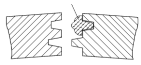
Разрез В-В: уплотняющая кромка EPDM
